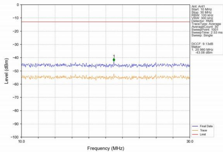
GSM850_GSM_LCH_824.2MHz_GSM_NTNV
