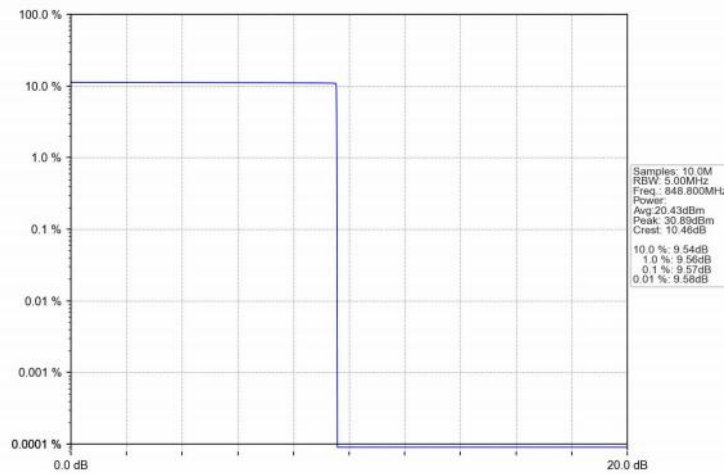
GSM850_GSM_HCH_848.8MHz_GSM_NTNV
