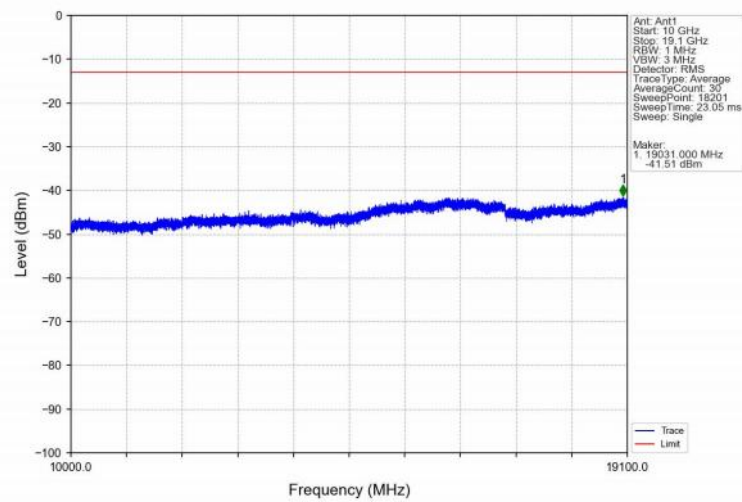
Band2_10MHz_QPSK_MCH_1880MHz_RB_1_0_NTNV
