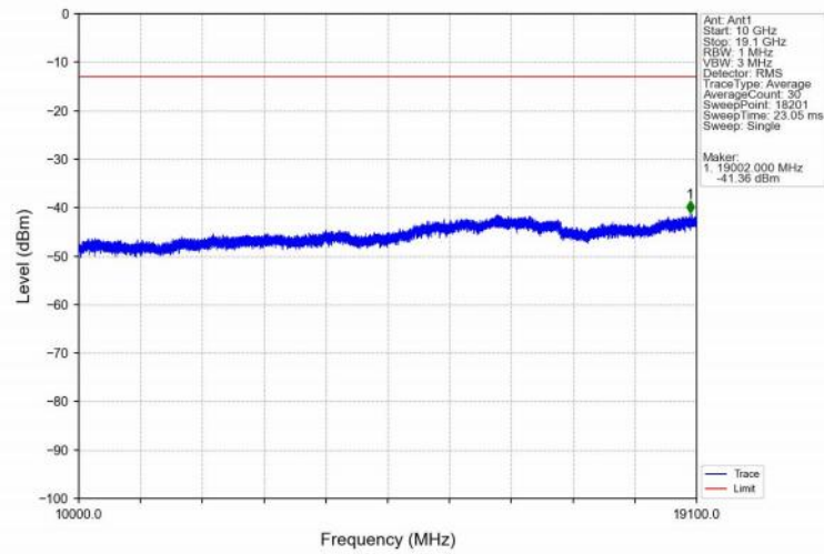
Band2_10MHz_16QAM_HCH_1905MHz_RB_1_49_NTNV
