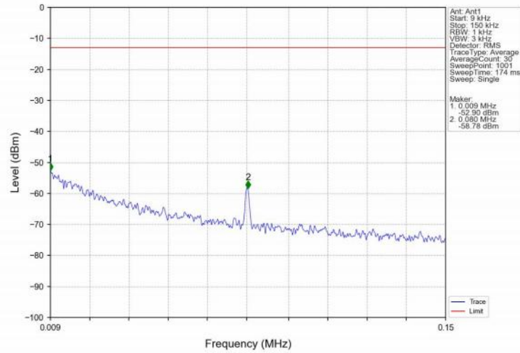
Band2_3MHz_16QAM_MCH_1880MHz_RB_1_0_NTNV
