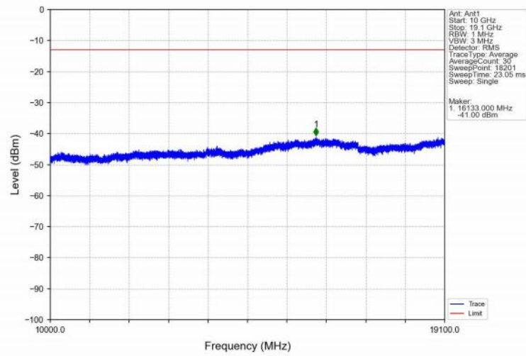
Band2_20MHz_QPSK_LCH_1860MHz_RB_1_0_NTNV
