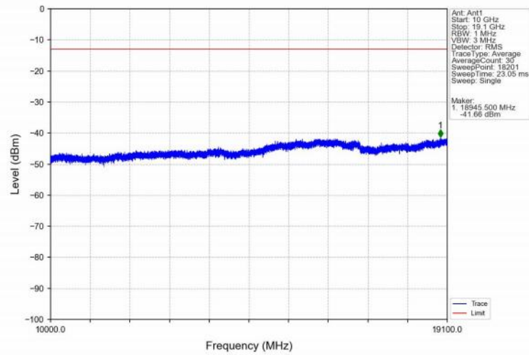
Band2_20MHz_QPSK_HCH_1900MHz_RB_1_99_NTNV
