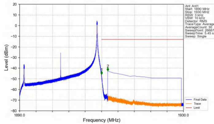
Band2_20MHz_16QAM_HCH_1900MHz_RB_1_99_NTNV
