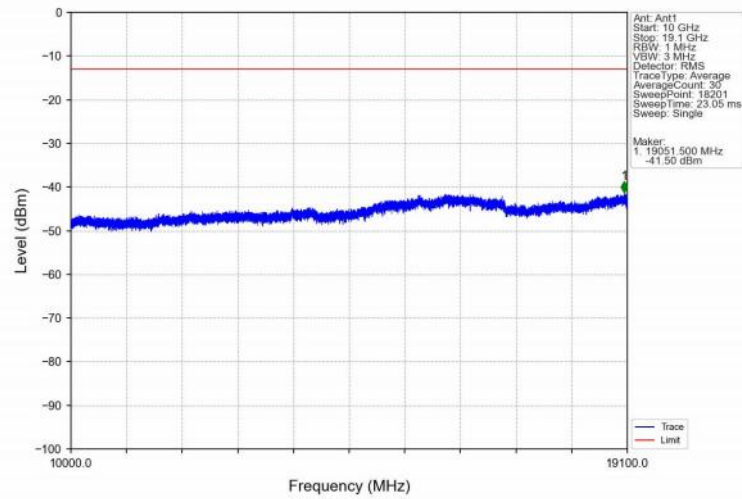
Band2_20MHz_16QAM_HCH_1900MHz_RB_1_99_NTNV
