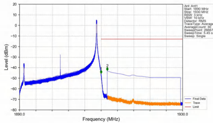
Band2_20MHz_QPSK_HCH_1900MHz_RB_1_99_NTNV
