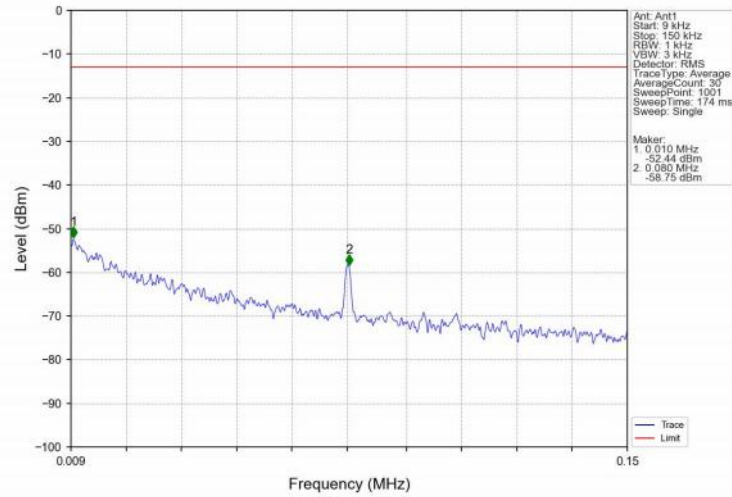
Band2_10MHz_16QAM_LCH_1855MHz_RB_1_0_NTNV
