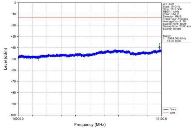
Band2_10MHz_QPSK_HCH_1905MHz_RB_1_49_NTNV
