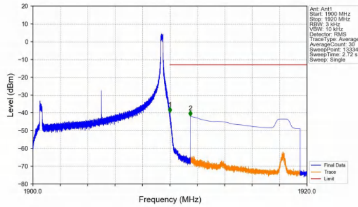
Band2_10MHz_16QAM_HCH_1905MHz_RB_1_49_NTNV
