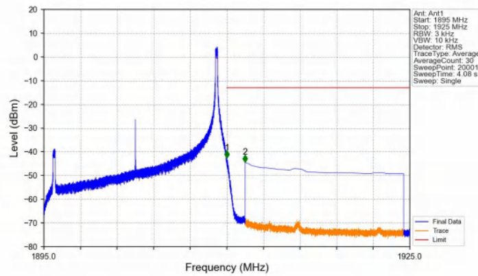
Band2_15MHz_16QAM_HCH_1902.5MHz_RB_1_74_NTNV
