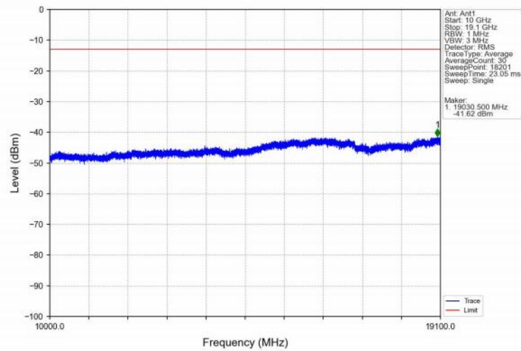
Band2_5MHz_QPSK_MCH_1880MHz_RB_1_0_NTNV
