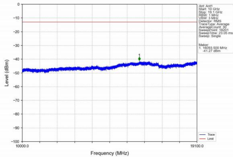
Band2_15MHz_QPSK_MCH_1880MHz_RB_1_0_NTNV
