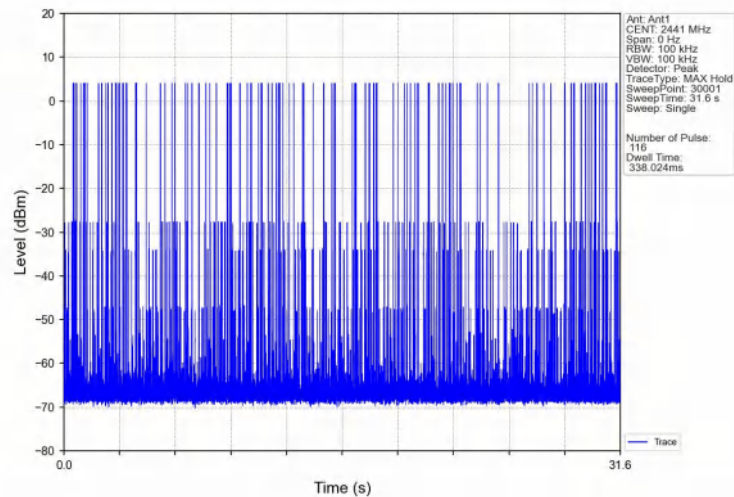
GFSK_DH5_HOPP_Ant1_NTNV
