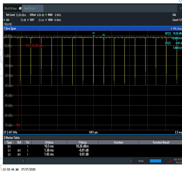
NTNV-11G-Ant0-2437
