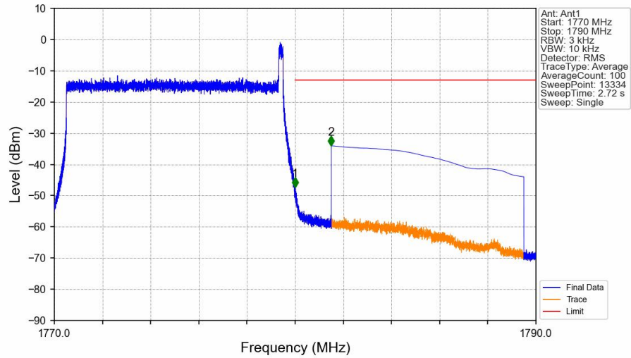
Band66_10MHz_QPSK_HCH_1775MHz_RB_1_49_NTNV
