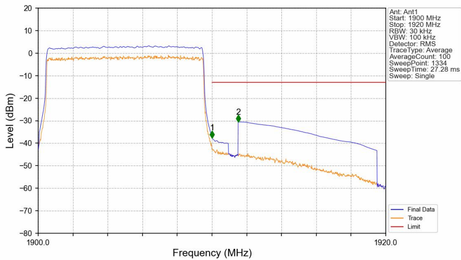
Band2_10MHz_QPSK_HCH_1905MHz_RB_50_0_NTNV
