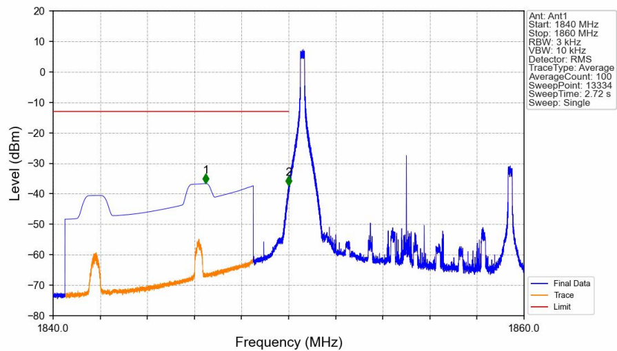
Band2_10MHz_16QAM_LCH_1855MHz_RB_1_0_NTNV
