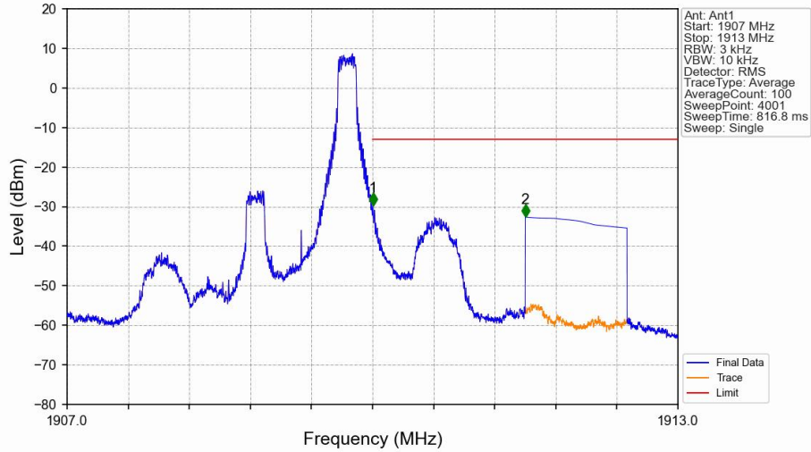
Band2_1.4MHz_QPSK_HCH_1909.3MHz_RB_1_5_NTNV
