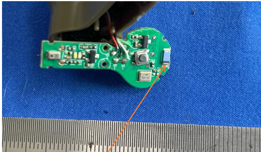
Antenna
