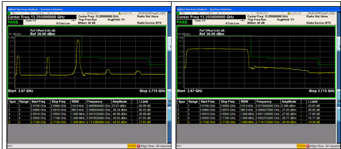
Band41_20MHz_QPSK_41490_1RB#99
