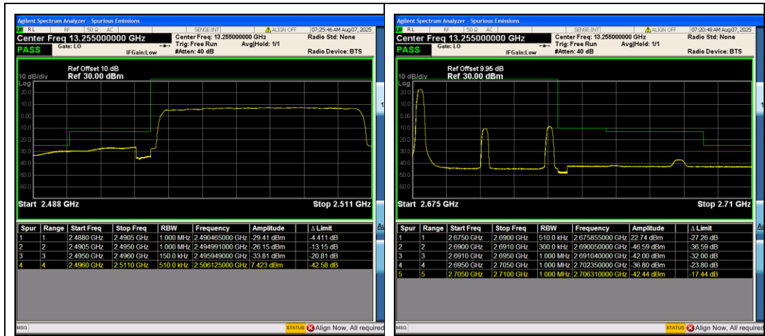
Band41_15MHz_QPSK_39725_75RB#0
