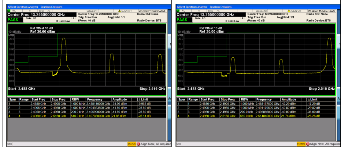
Band41_20MHz_QPSK_41490_1RB#99
