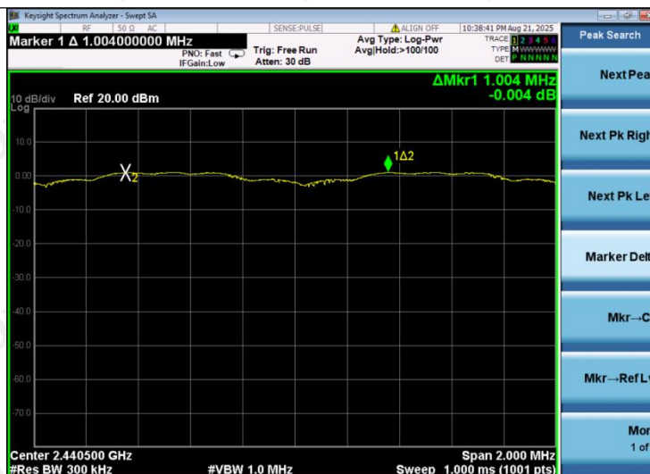
\pi/4 DQPSK
