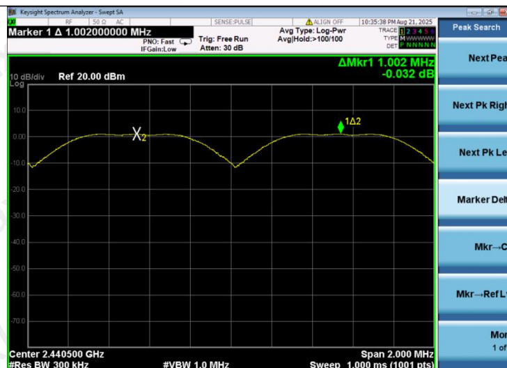
GFSK
