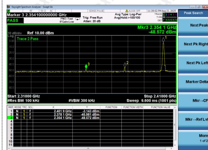
Left Band edge hoping off
