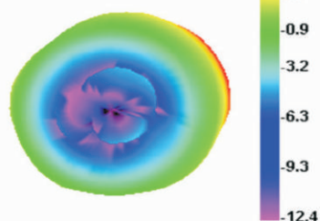
2450.000MHz E1
