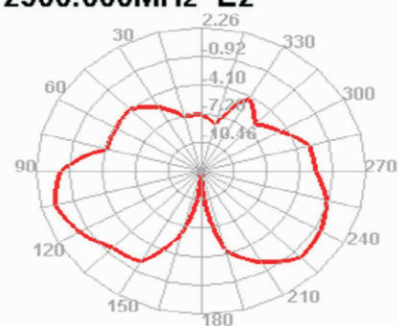
2500.000MHz E2
