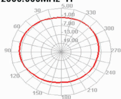
2500.000MHz H
