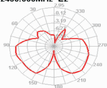
2450.000MHz E2
