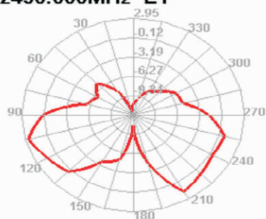
2450.000MHz E1
