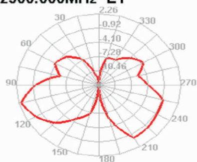
2500.000MHz E1
