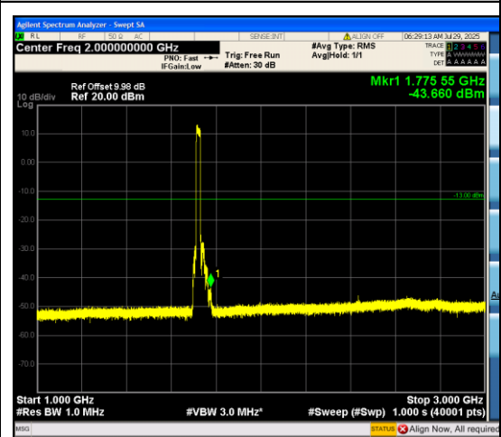
Band66_20MHz_QPSK_132072_100RB#0_100 0~3000_1000~3000
