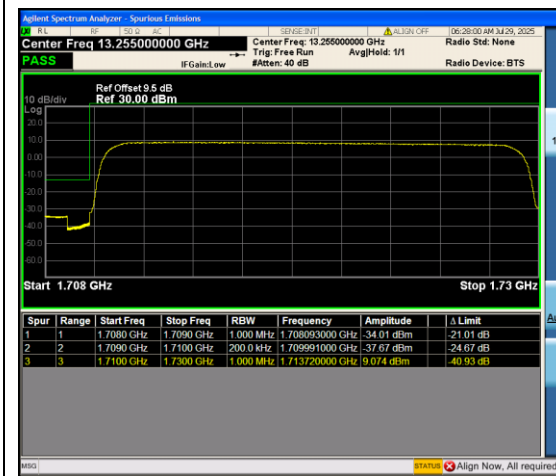
Band66_20MHz_QPSK_132072_100RB#0
