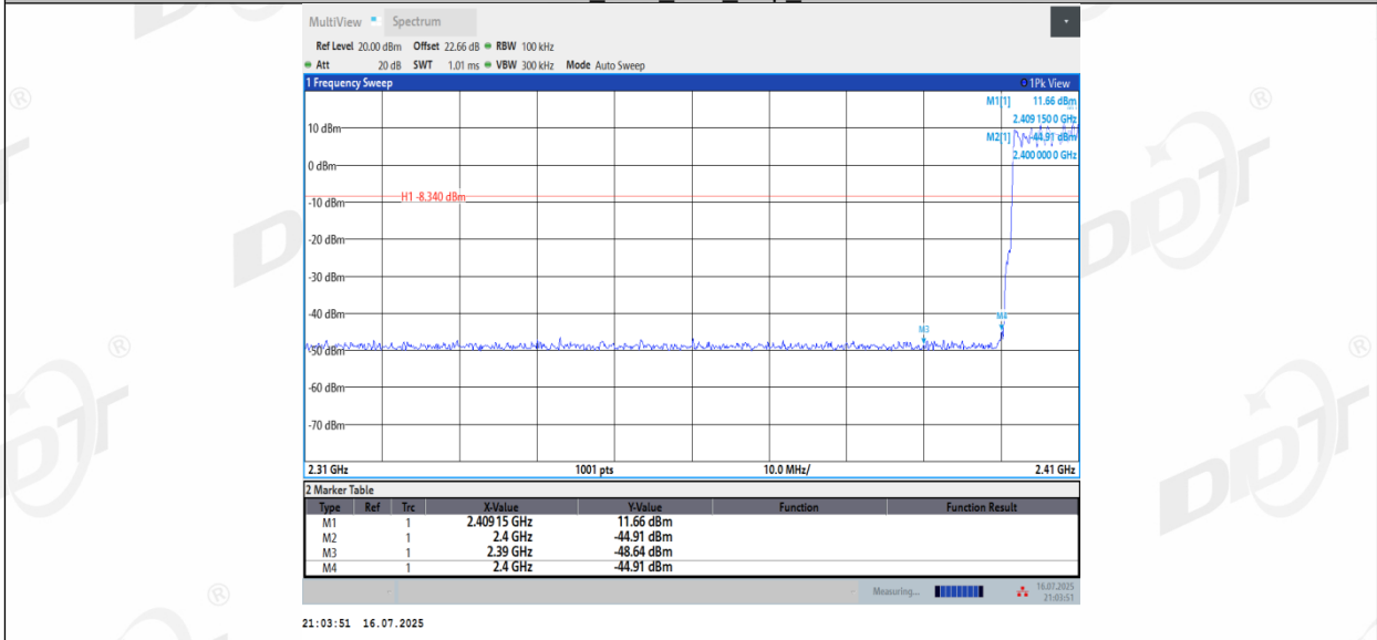
3DH5_Ant2_Low_Hop_2402
