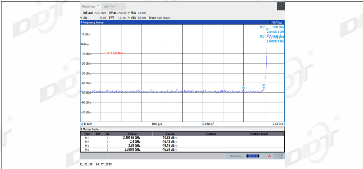
2DH5_Ant2_Low_Hop_2402
