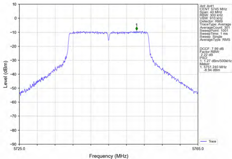
802.11n(HT20)_LCH_5745MHz_Ant1_NTNV
