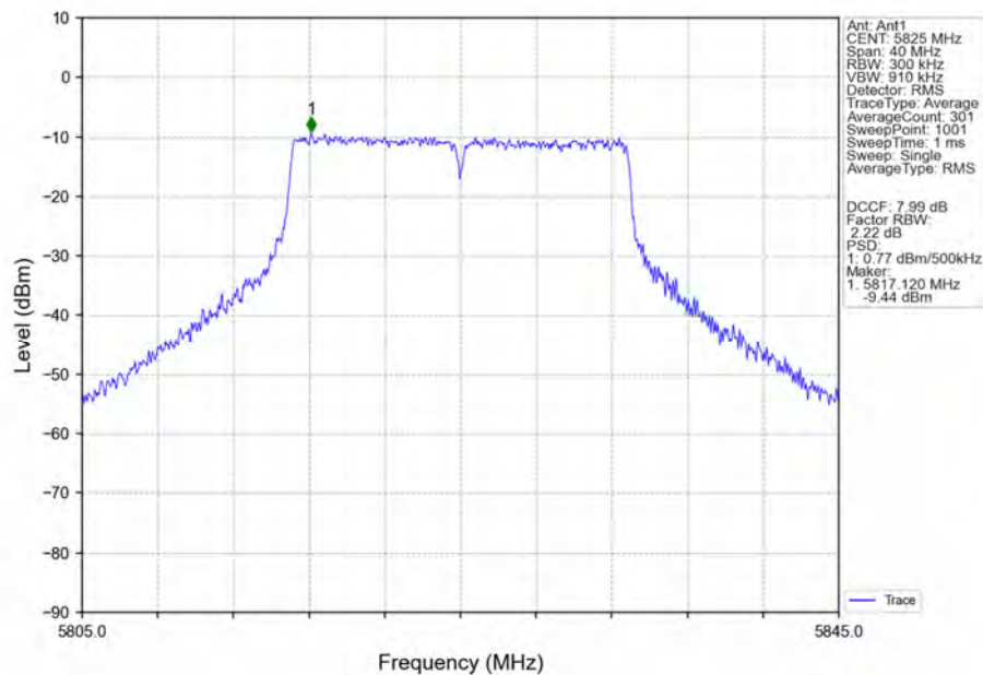
802.11n(HT20)_HCH 5825MHz_Ant1_NTNV
