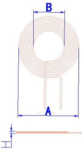
图一、线圈
