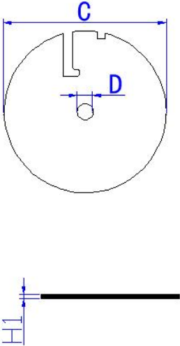
图二、磁片
