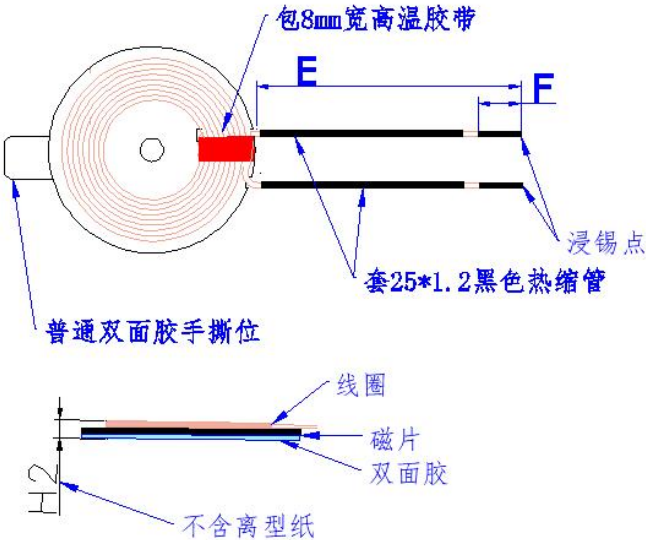
图三、线圈与磁片组合
