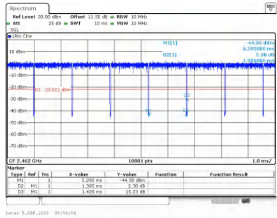
IEEE 802.11g_20MHz_Channel 11
