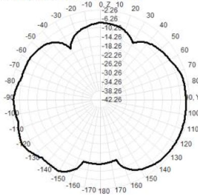
2500.0MHz Total(E2-YZ), Max=-2.26dBi
