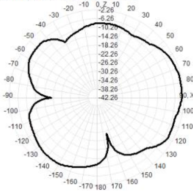
2500.0MHz Total(E1-XZ), Max=-3.38dBi
