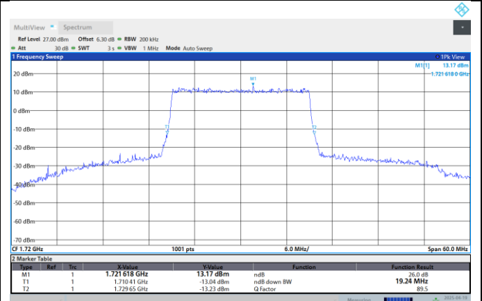
Band66-20MHz-QPSK-132572-100RB#0
