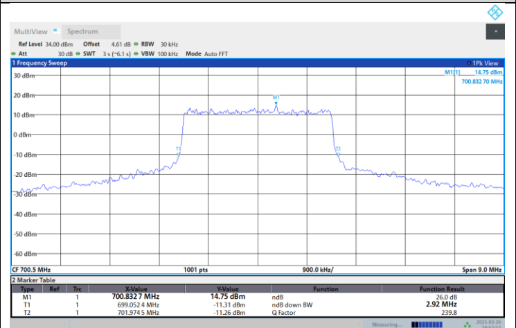
Band12-3MHz-QPSK-23165-15RB#0
