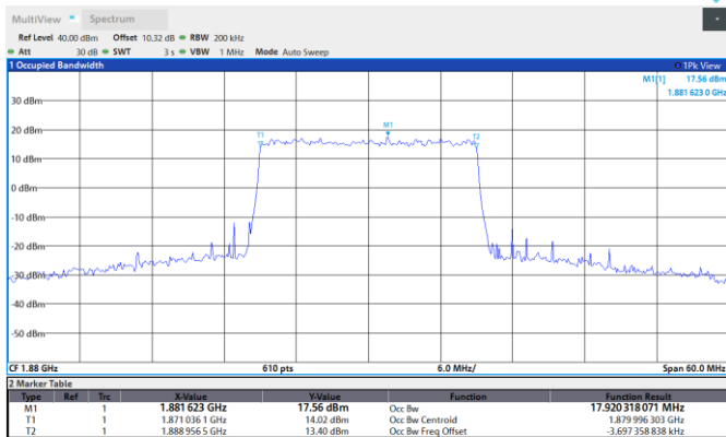
Band2-20MHz-16QAM-18700-100RB#0
