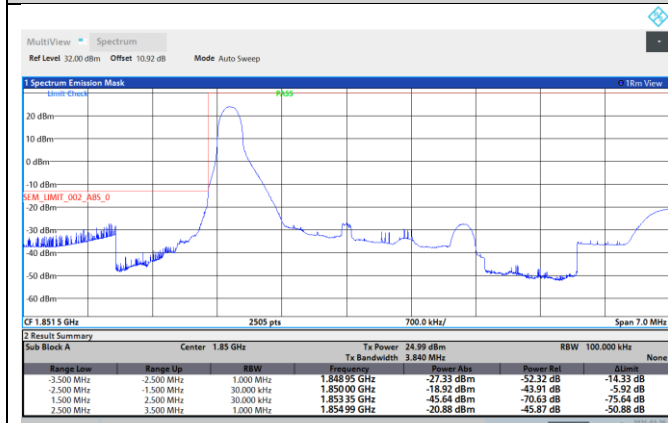
Band2-3MHz-QPSK-18615-1RB#0
