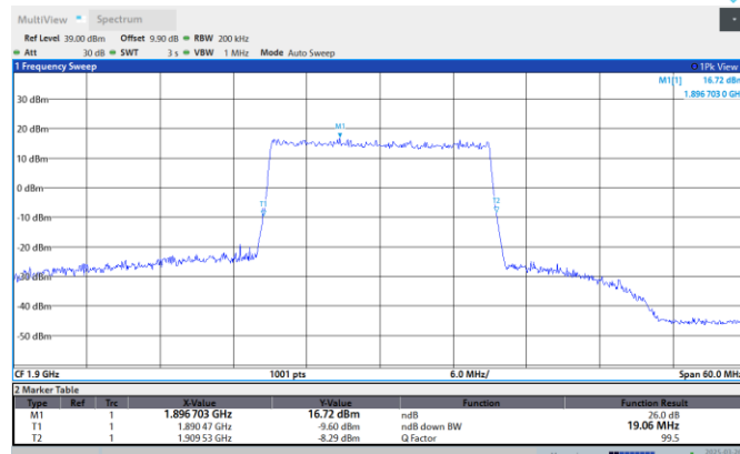
Band2-20MHz-16QAM-18900-100RB#0
