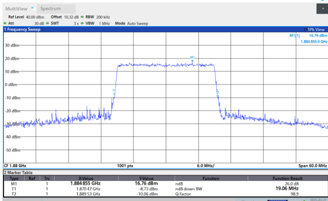
Band2-20MHz-16QAM-18700-100RB#0
