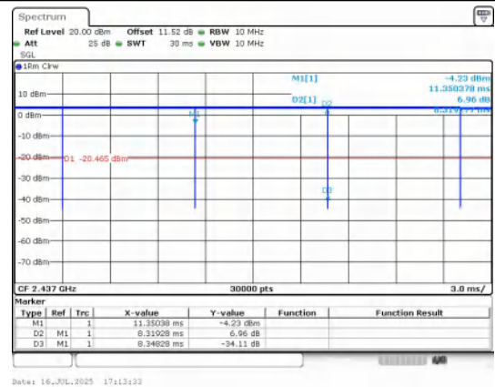
IEEE 802.11b_20MHz_Channel 6
