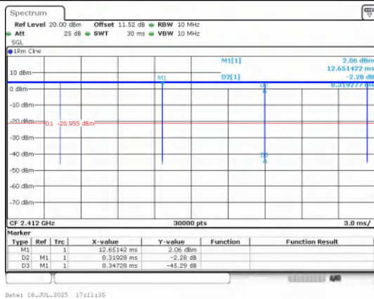
IEEE 802.11b_20MHz_Channel 1
