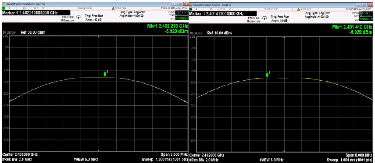
2402MHz(1Mbps)
