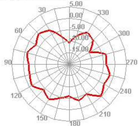
2400.000MHz E2
