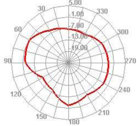
2400.000MHz H
