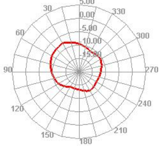
2400.000MHz H
