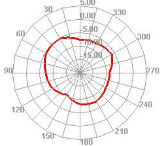
2450.000MHz H
