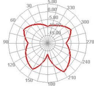
2450.000MHz E1
