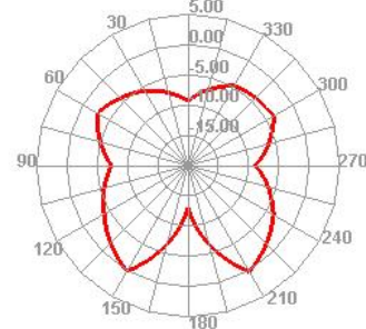
2450.000MHz E2
