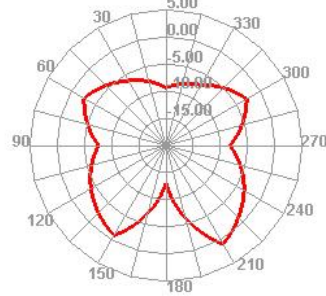
2450.000MHz E1
