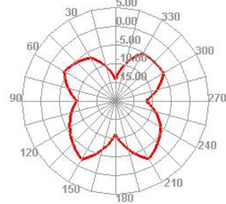
2400.000MHz E2
