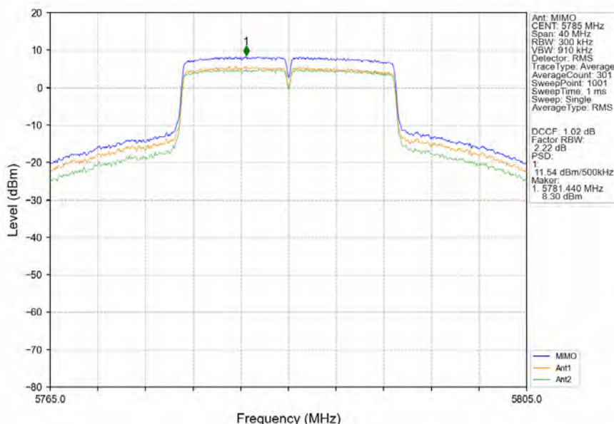
802.11n(HT20)_MCH_5785MHz_MIMO_NTNV
