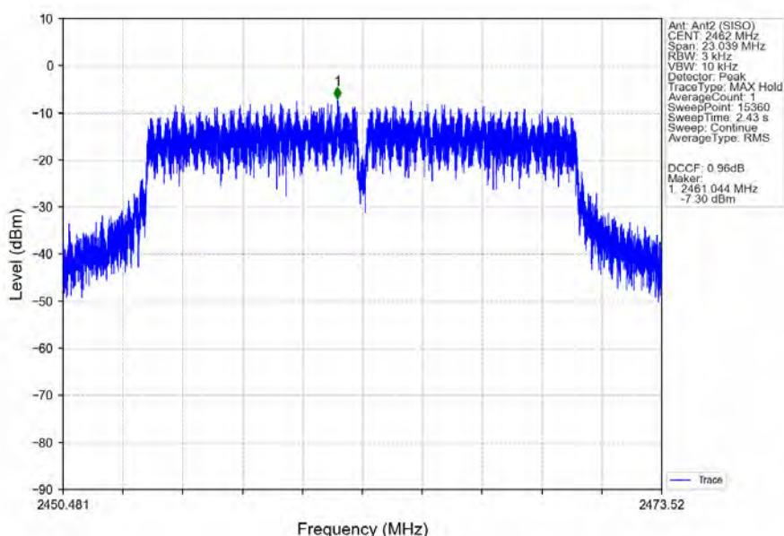
802.11g_HCH_2462MHz_Ant2 (SISO)_NTNV
