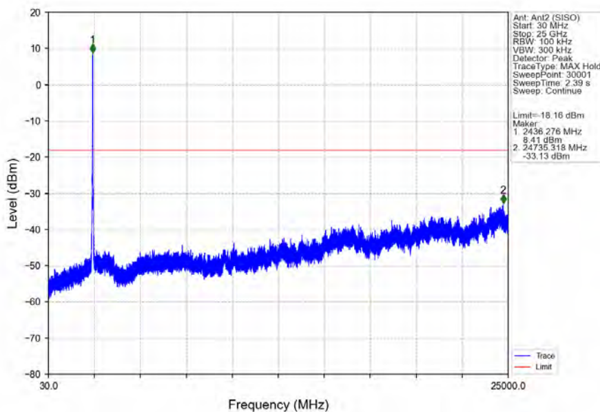
802.11g_MCH_2437MHz_Ant2 (SISO)_NTNV
