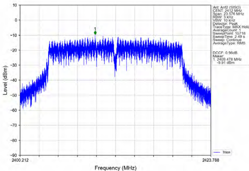
802.11g_LCH_2412MHz_Ant2 (SISO)_NTNV
