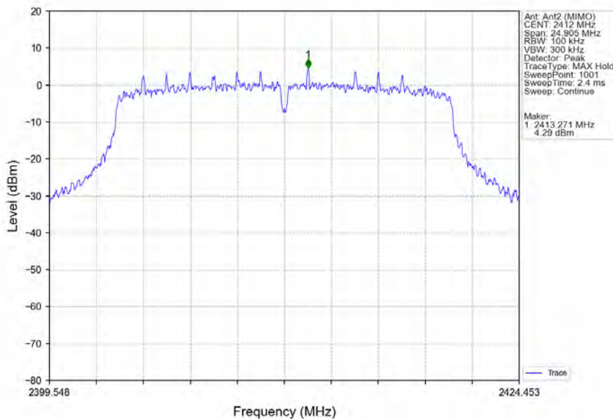
802.11n(HT20)_LCH_2412MHz_Ant2 (MIMO)_NTNV
