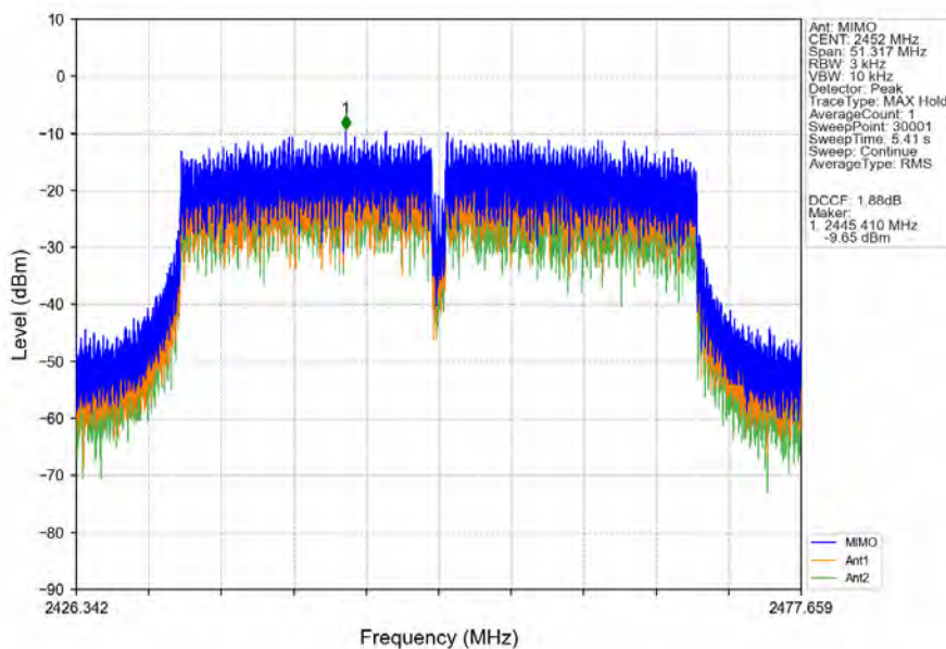
802.11n(HT40)_HCH_2452MHz_MIMO_NTNV
