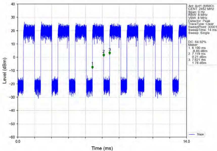
802.11n(HT40)_HCH_2452MHz_Ant1 (MIMO)_NTNV
