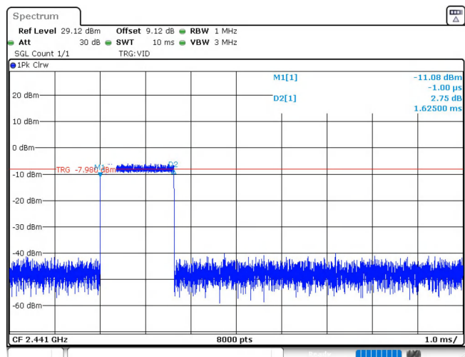
3DH3_Ant1_Hop
