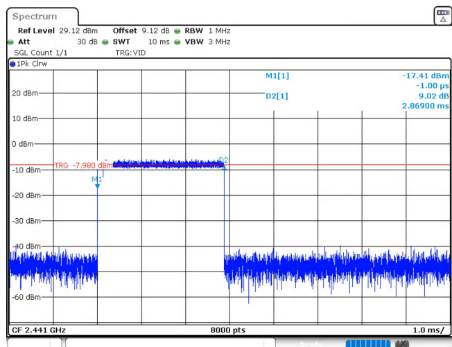
3DH5_Ant1_Hop
