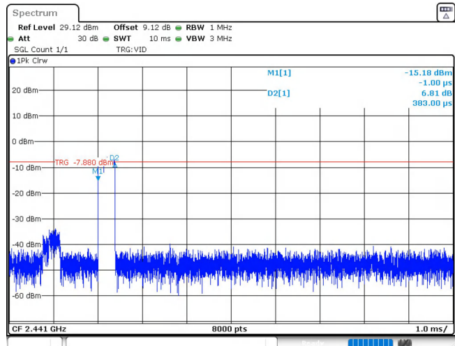
3DH1_Ant1_Hop
