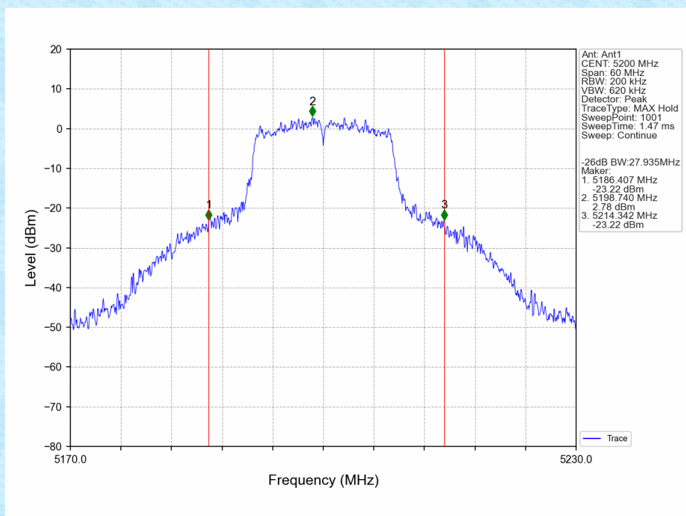
802.11a_MCH_5200MHz_Ant1_NTNV
