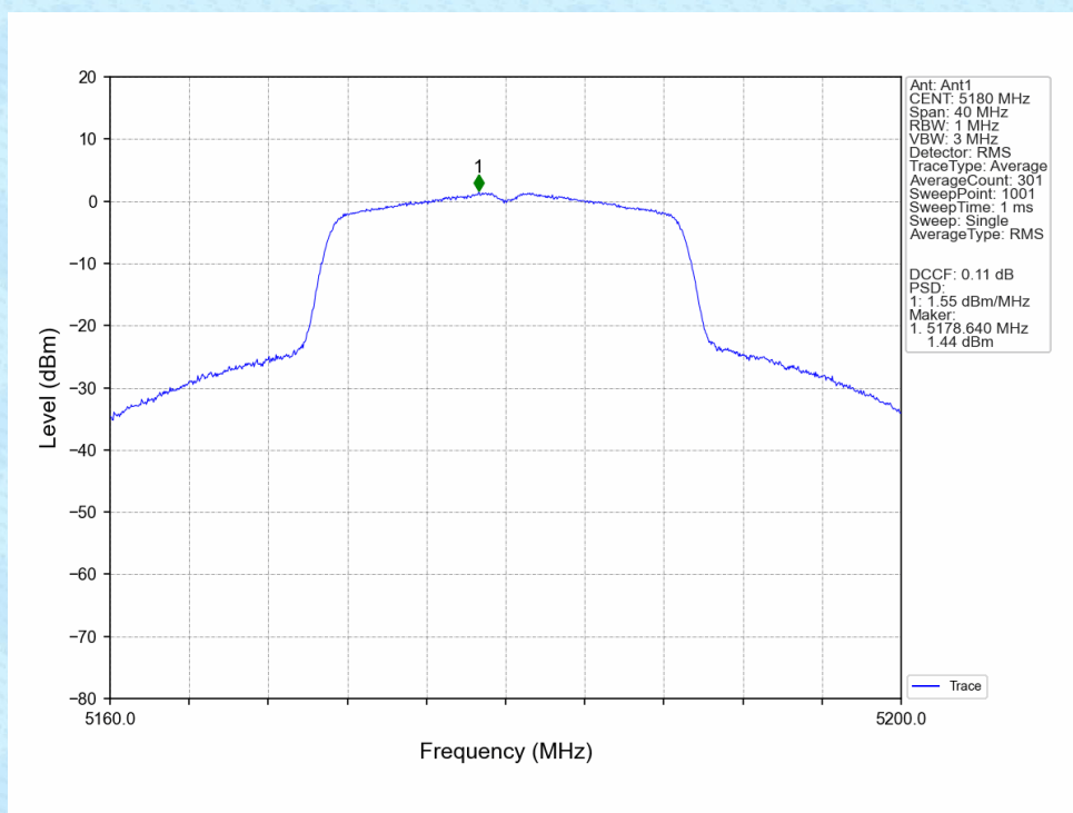
802.11n(HT20)_LCH_5180MHz_Ant1_NTNV
