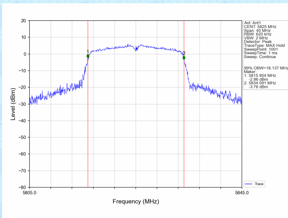
802.11n(HT20)_HCH_5825MHz_Ant1_NTNV
