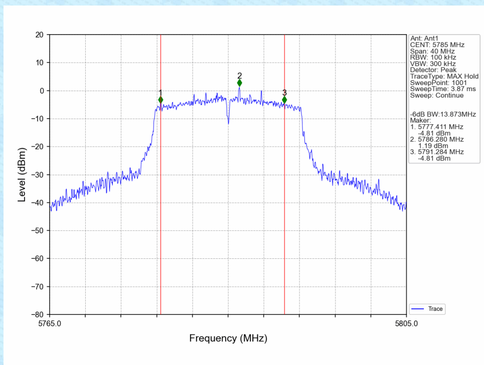
802.11a_MCH_5785MHz_Ant1_NTNV
