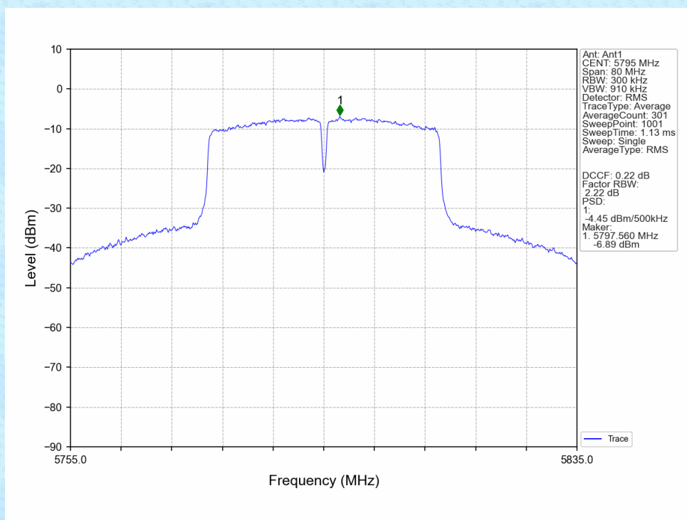
802.11n(HT40)_HCH_5795MHz_Ant1_NTNV
