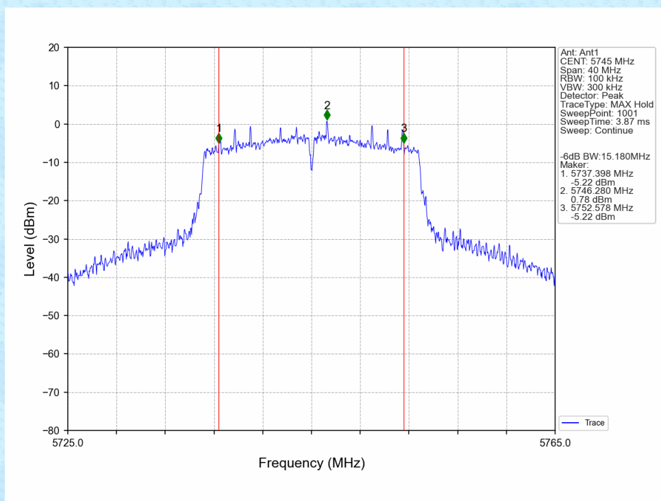
802.11n(HT20)_LCH_5745MHz_Ant1_NTNV
