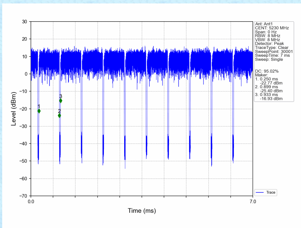
802.11n(HT40)_HCH_5230MHz_Ant1_NTNV
