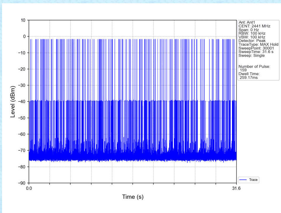
GFSK_DH3_HOPP_Ant1_NTNV
