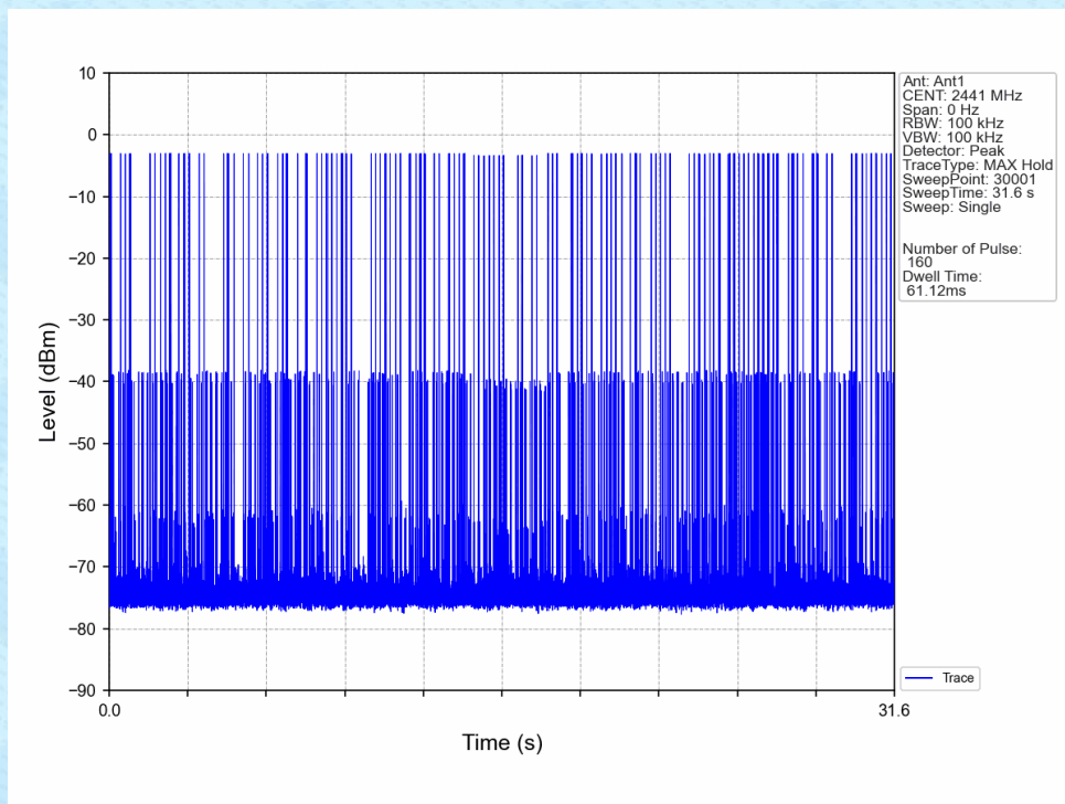
Pi/4DQPSK_2DH3_HOPP_Ant1_NTNV
