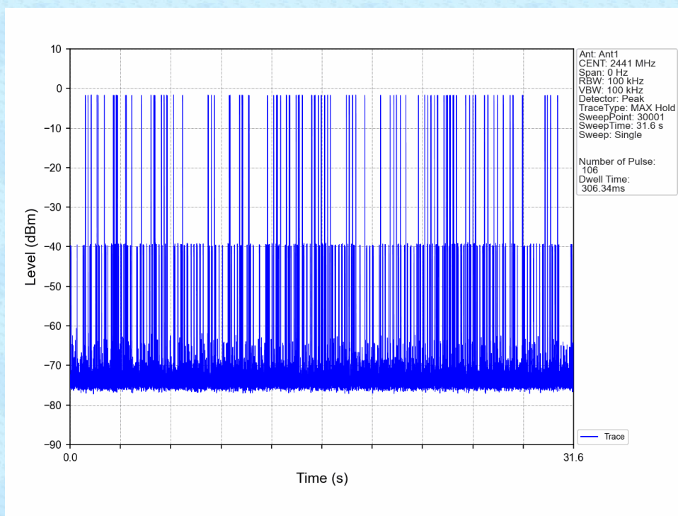
GFSK_DH5_HOPP_Ant1_NTNV
