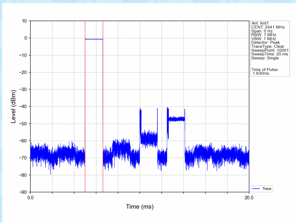
GFSK_DH3_HOPP_Ant1_NTNV
