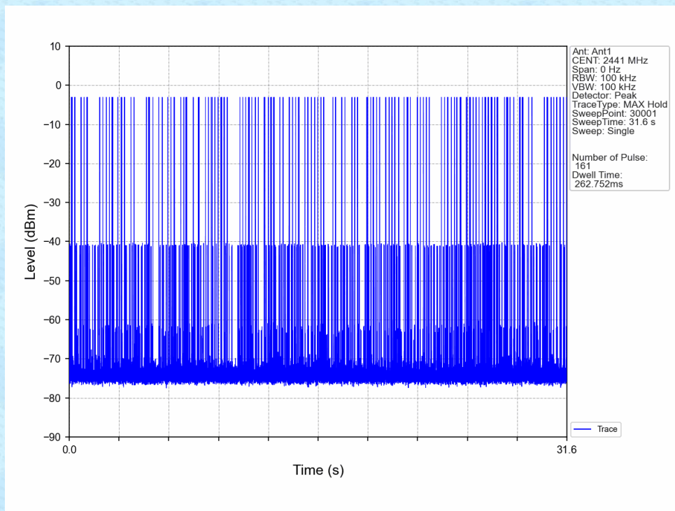
8DPSK_3DH3_HOPP_Ant1_NTNV
