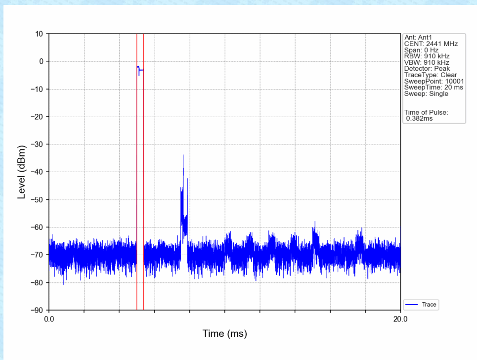
Pi/4DQPSK_2DH1_HOPP_Ant1_NTNV
