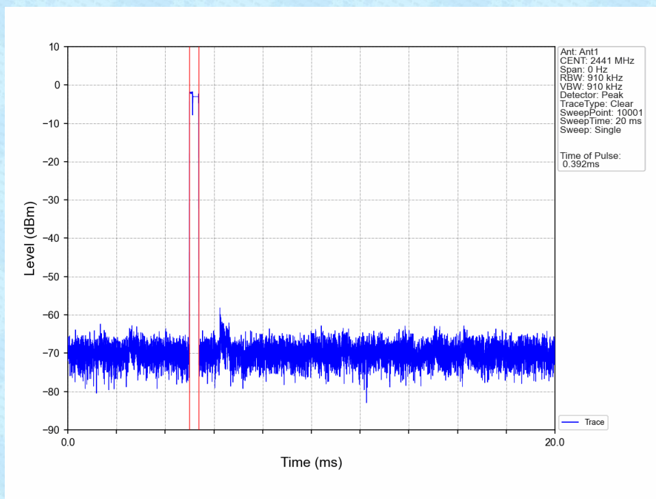
8DPSK_3DH1_HOPP_Ant1_NTNV
