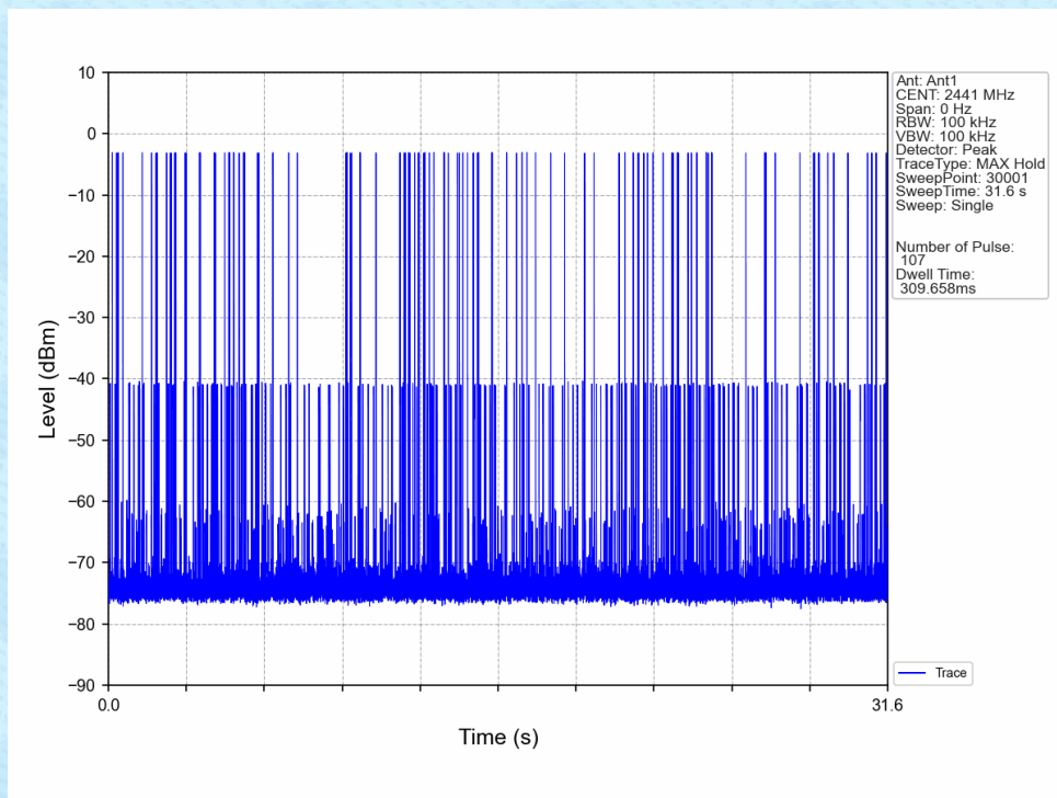
8DPSK_3DH5_HOPP_Ant1_NTNV
