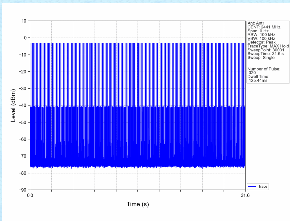
8DPSK_3DH1_HOPP_Ant1_NTNV
