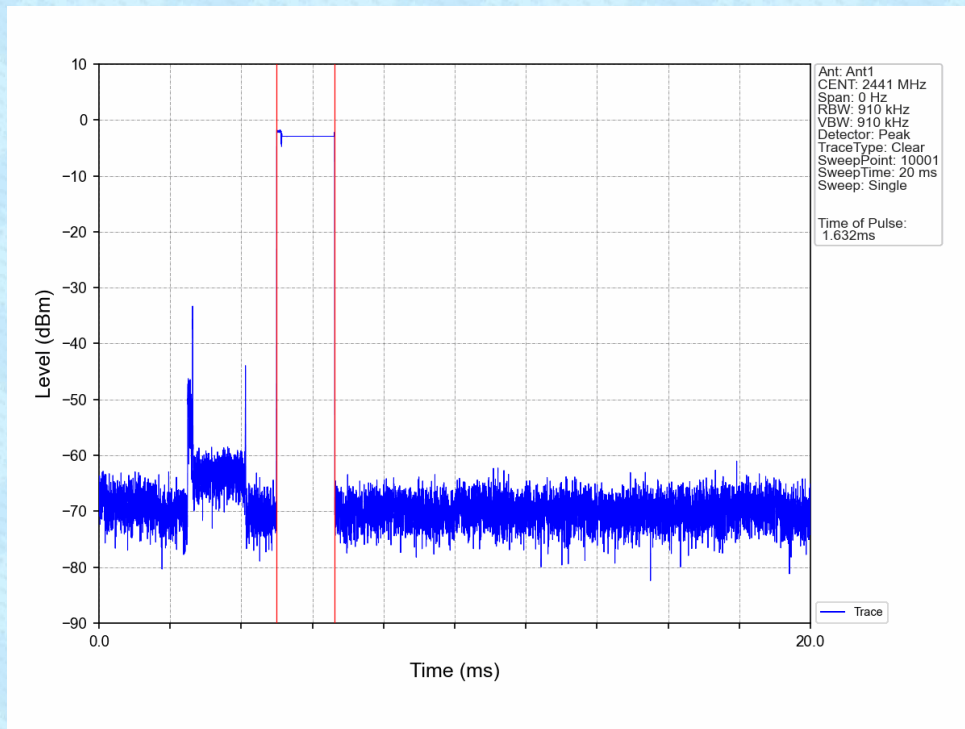
8DPSK_3DH3_HOPP_Ant1_NTNV
