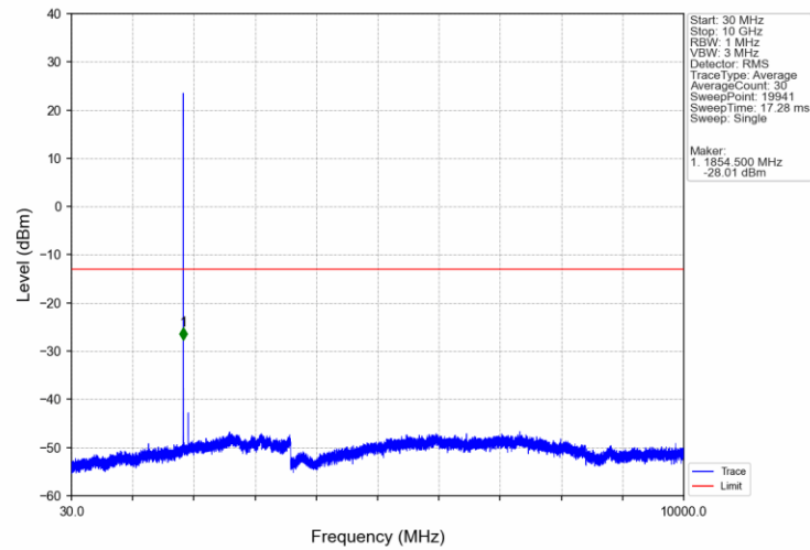
Band2 1.4MHz QPSK LCH 1850.7MHz RB 1 0 NTNV
