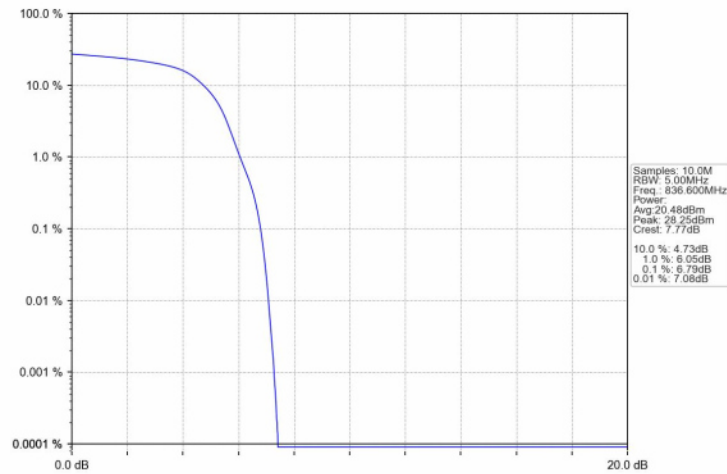
Band5_HSUPA_MCH_836.6MHz_Subtest 1_NTNV
