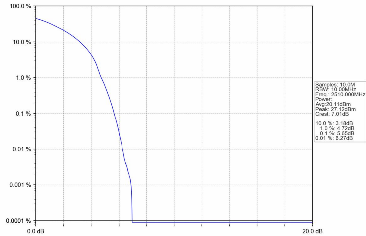
Band7_20MHz_QPSK_LCH_2510MHz_RB_100_0_NTNV
