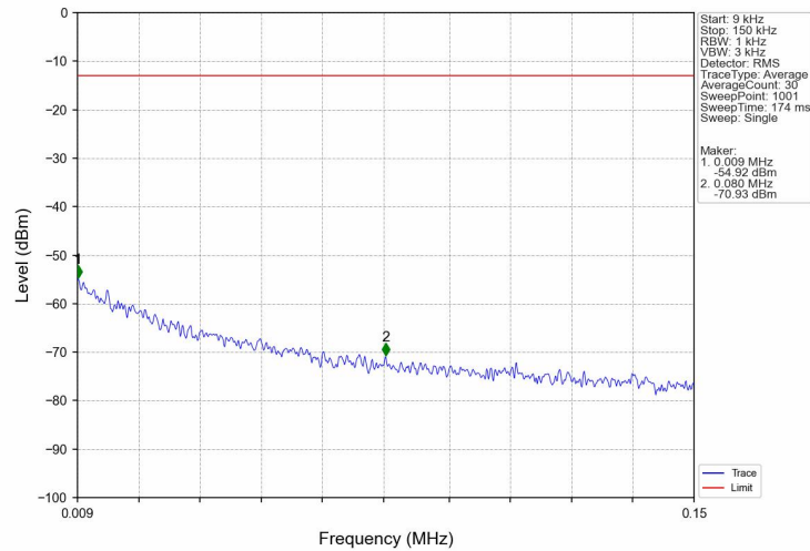
Band5_10MHz_QPSK_LCH_829MHz_RB_1_0_NTNV
