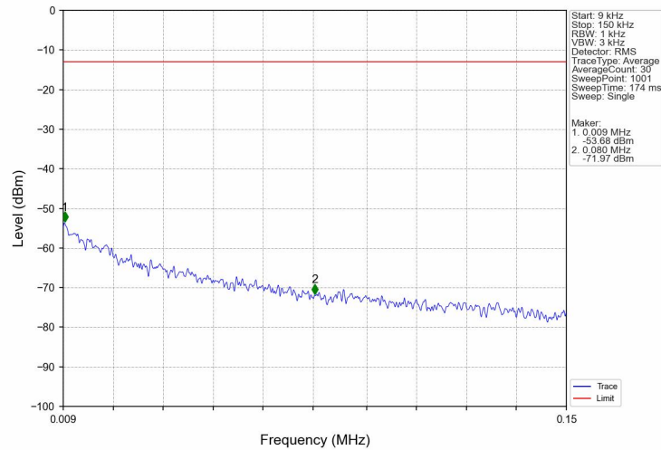
Band4_20MHz_QPSK_LCH_1720MHz_RB_1_0_NTNV
