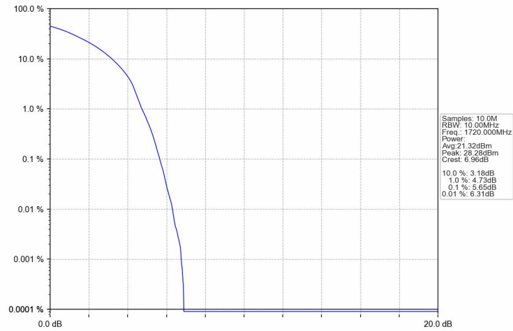
Band4_20MHz_QPSK_LCH_1720MHz_RB_100_0_NTNV
