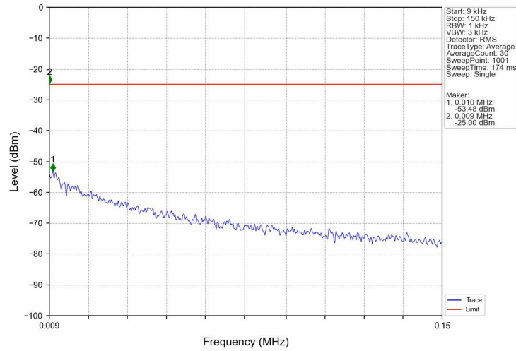
Band7_10MHz_QPSK_MCH_2535MHz_RB_1_0_NTNV
