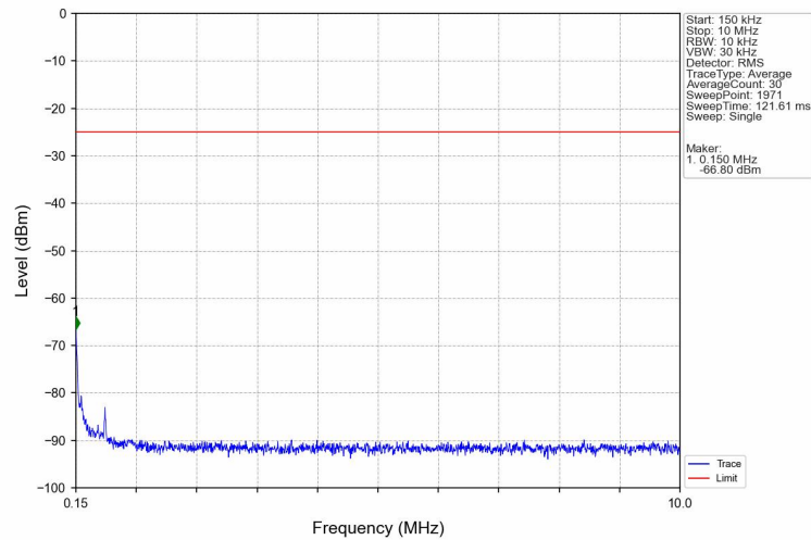
Band7_10MHz_QPSK_MCH_2535MHz_RB_1_0_NTNV
