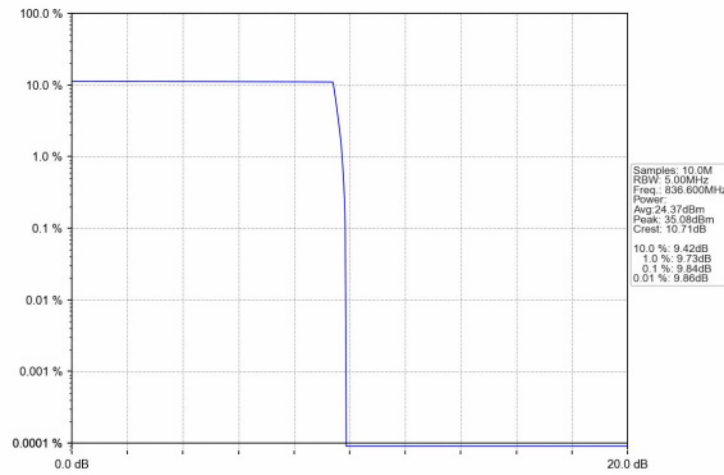
GSM850_GSM_MCH_836.6MHz_GSM_NTNV
