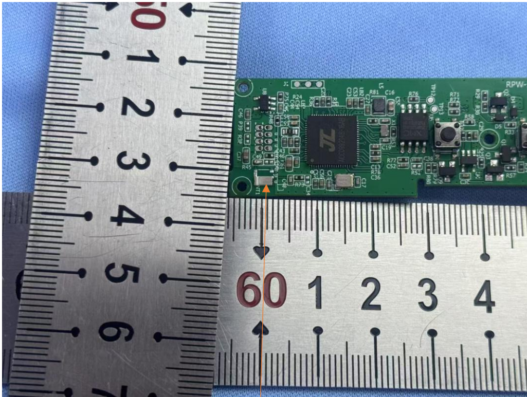
BT/WIFI ANT
