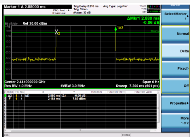
GFSK DH5
