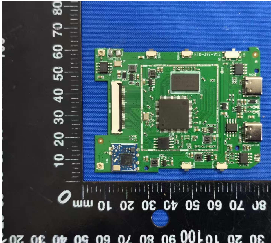
EUT Photo 9
