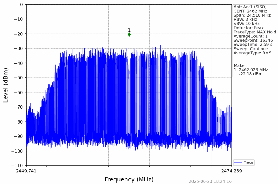
802.11g_HCH_2462MHz_Ant1 (SISO)_NTNV
