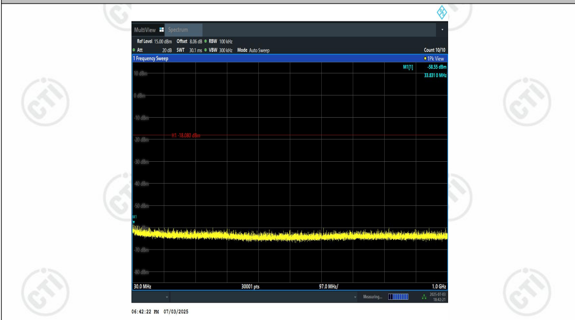
BLE_2M-Ant1-2440-30~1000-PASS
