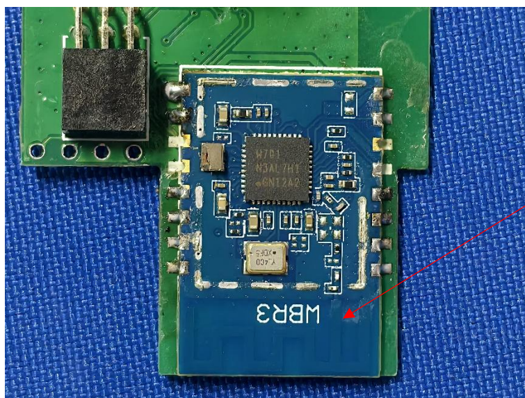
BT/WIFI ANT
