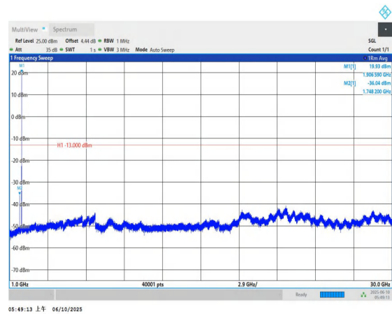
Band2-9538-1000~30000MHz-PASS
