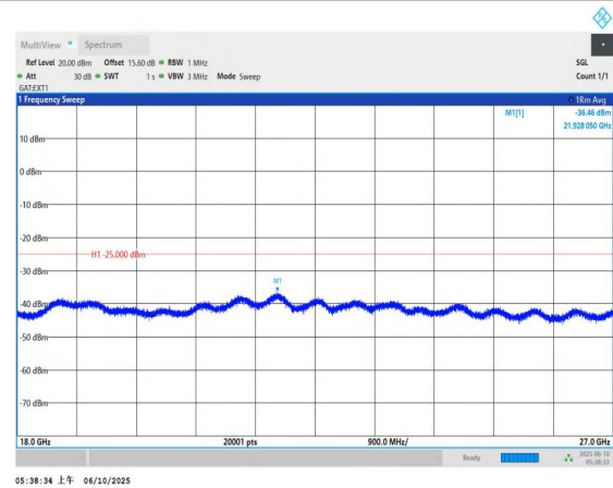
Band41-20MHz-QPSK-41490-1RB#0-18000~27000-PASS
