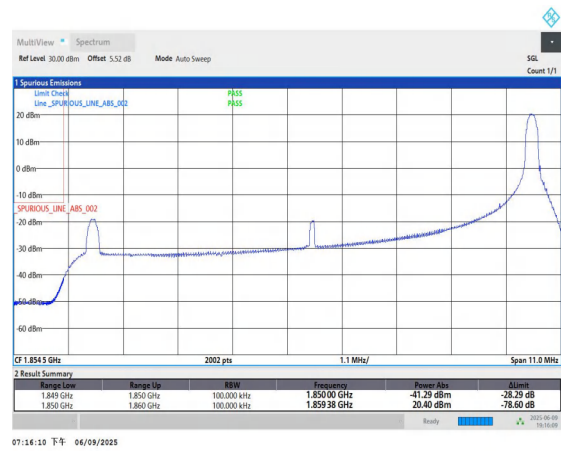
Band2-10MHz-QPSK-18650-1RB#49-PASS
