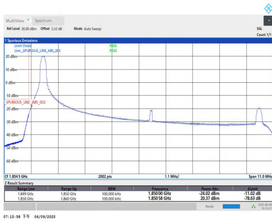
Band2-10MHz-QPSK-18650-1RB#0-PASS
