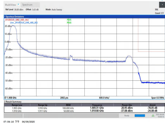
Band2-5MHz-QPSK-19175-1RB#0-PASS
