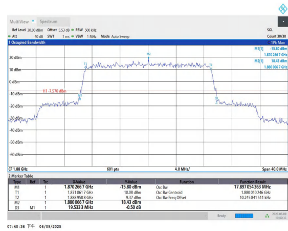
Band2-20MHz-QPSK-18900-100RB#0-PASS
