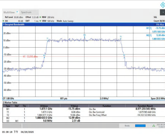
Band2-10MHz-16QAM-18900-50RB#0-PASS
