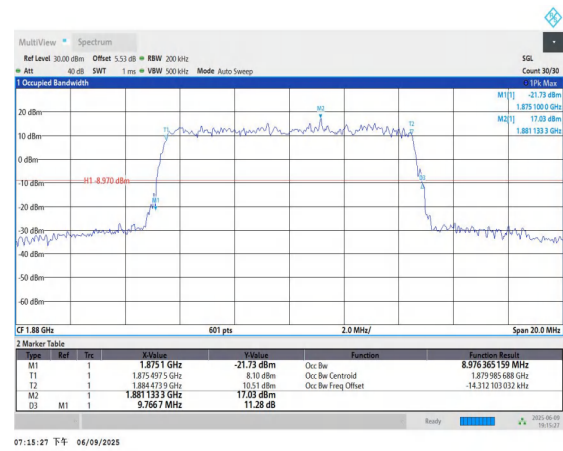
Band2-10MHz-QPSK-18900-50RB#0-PASS
