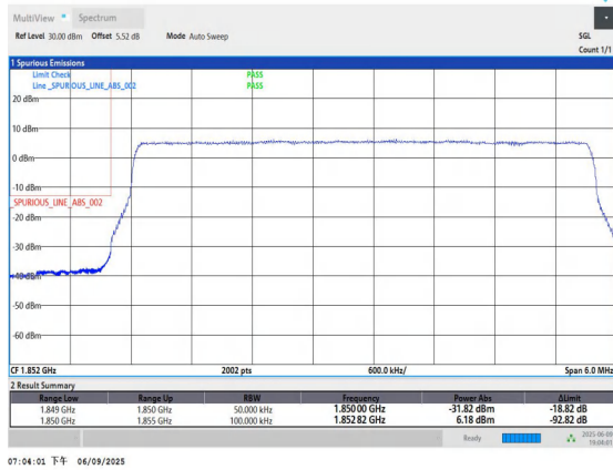
Band2-5MHz-QPSK-18625-25RB#0-PASS
