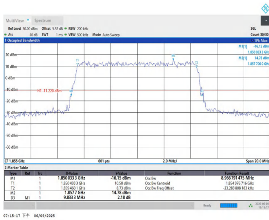
Band2-10MHz-QPSK-18650-50RB#0-PASS
