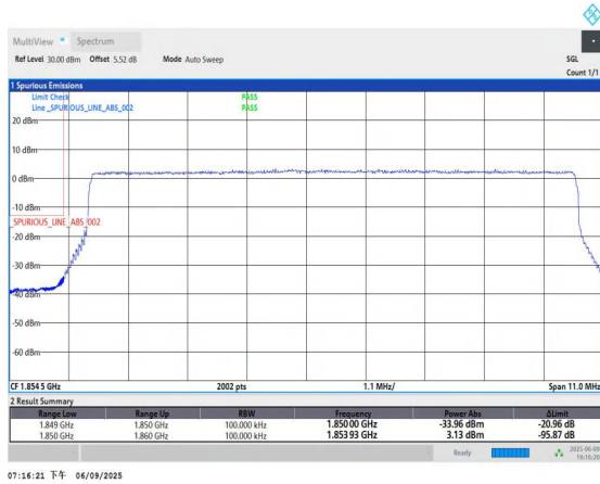
Band2-10MHz-QPSK-18650-50RB#0-PASS
