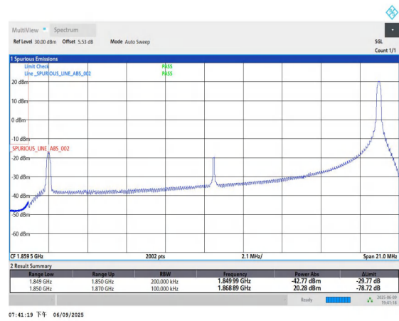
Band2-20MHz-QPSK-18700-1RB#99-PASS
