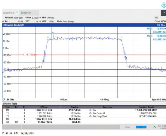
Band2-20MHz-QPSK-18700-100RB#0-PASS
