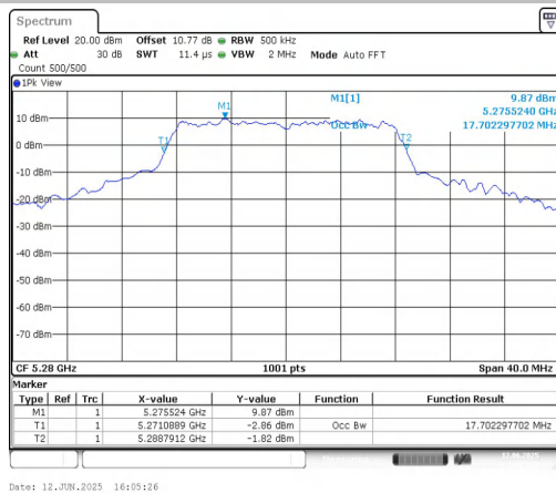
11A-Ant1-5280
