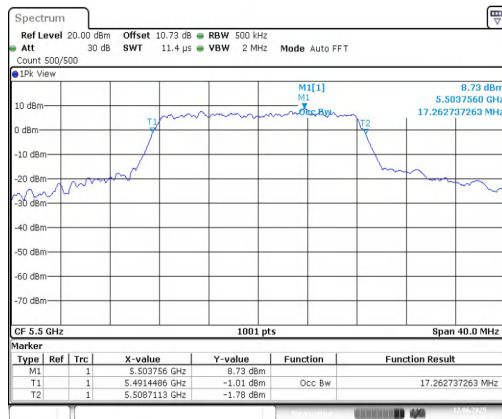
11A-Ant1-5500
