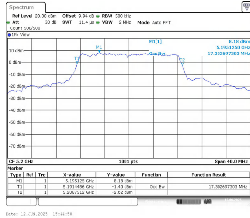
11A-Ant1-5200
