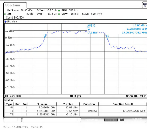
11A-Ant1-5260
