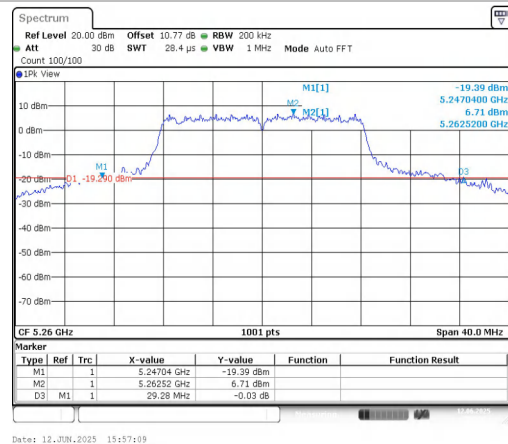
11A-Ant1-5260
