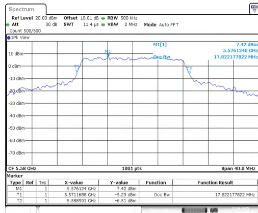
11A-Ant1-5580
