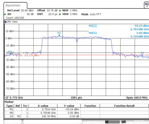
11AC80SISO-Ant1-5775
