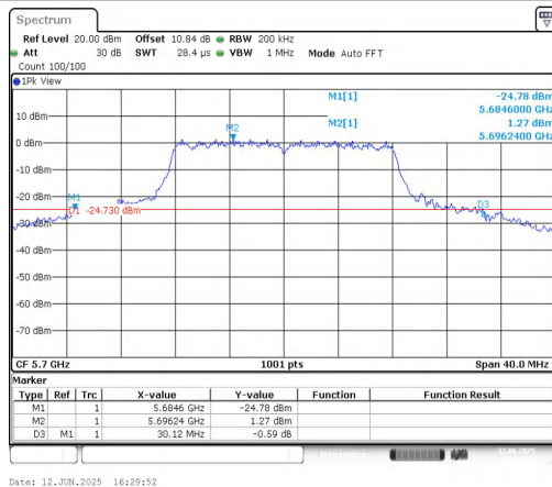
11A-Ant1-5700
