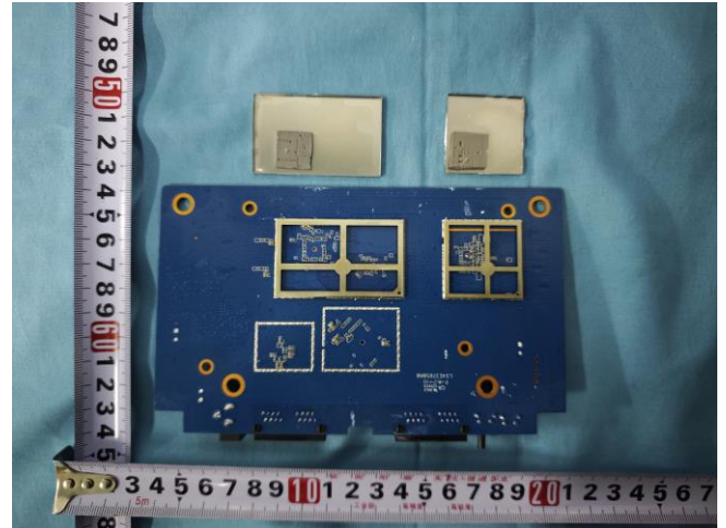
EUT 2
