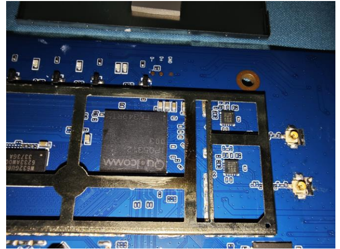
IC 2
