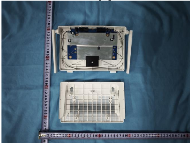
EUT 1
