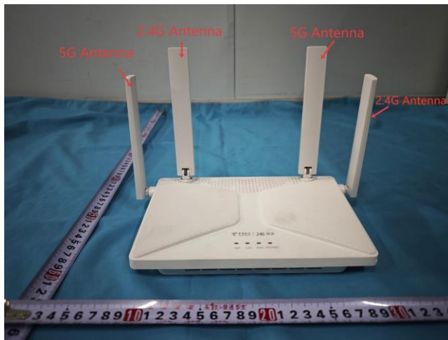
ANTENNA
